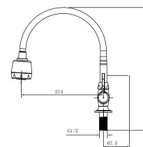
Ta-6973CP Vòi bếp đơn lạnh
