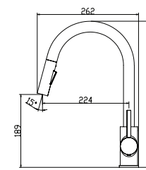
Ta-629PCP Vòi bếp ●
