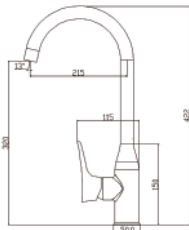
Ta-6443CP-2 Vòi bếp ●
