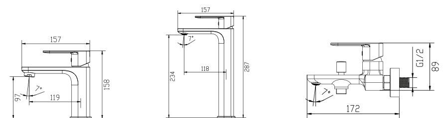
Ta-8071CP Vòi lavabo ●
