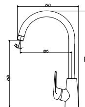
Ta-6353CP Vòi bếp ●
