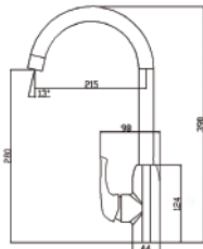
Ta-7923CP Vòi bếp ●
