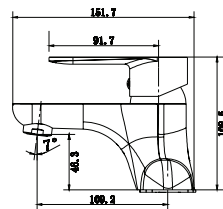
Ta-6132CP Vòi lavabo ●
