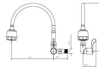
Ta-6973-2CP Vòi bếp đơn lạnh
