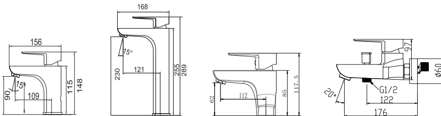
Ta-6261CP Vòi lavabo ●
