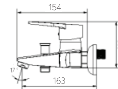
Ta-6044CP Sen tắm ●
