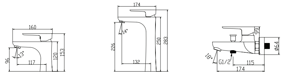
Ta-6311CP Vòi lavabo ●
