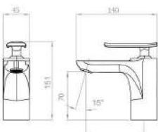
NEW HU-510 세면기 원홀 수전 Basin Mixer One-hole Giá: 3.100.000VNĐ
