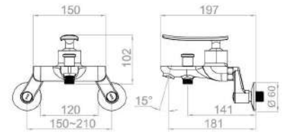
NEW HU-330N 세면기 원홀 수전 Basin Mixer One-hole Giá: 2.200.000VNĐ
