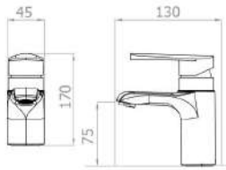
NEW HU-310N 세면기 원홀 수전 Basin Mixer One-hole Giá: 1.600.000VNĐ
