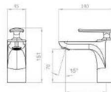
NEW HU-1110 세면기 원홀 수전 Basin Mixer One-hole Giá: 3.100.000VNĐ
