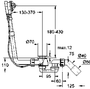
28 943 000 Talento pop-up waste
