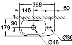
39 327 00H Mini handrinse basin, 37 cm
